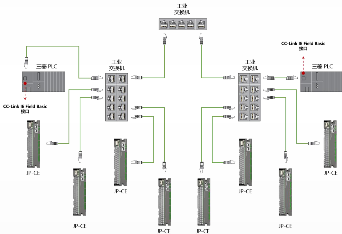
图 5-3 CC-Link IE Field Basic 树形网络拓扑结构
