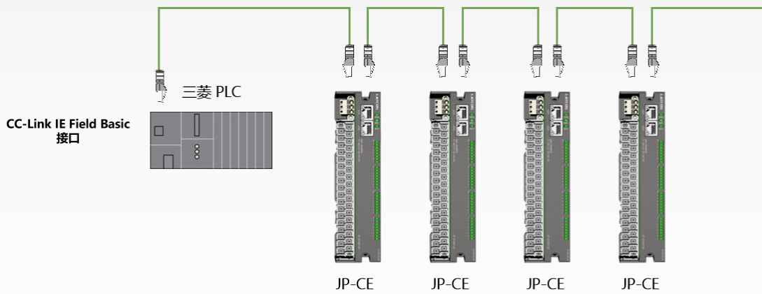
图 5-2 CC-Link IE Field Basic 菊花链路由拓扑结构
