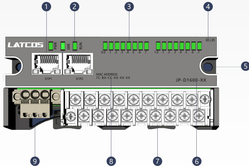
图 3 模块接线图
