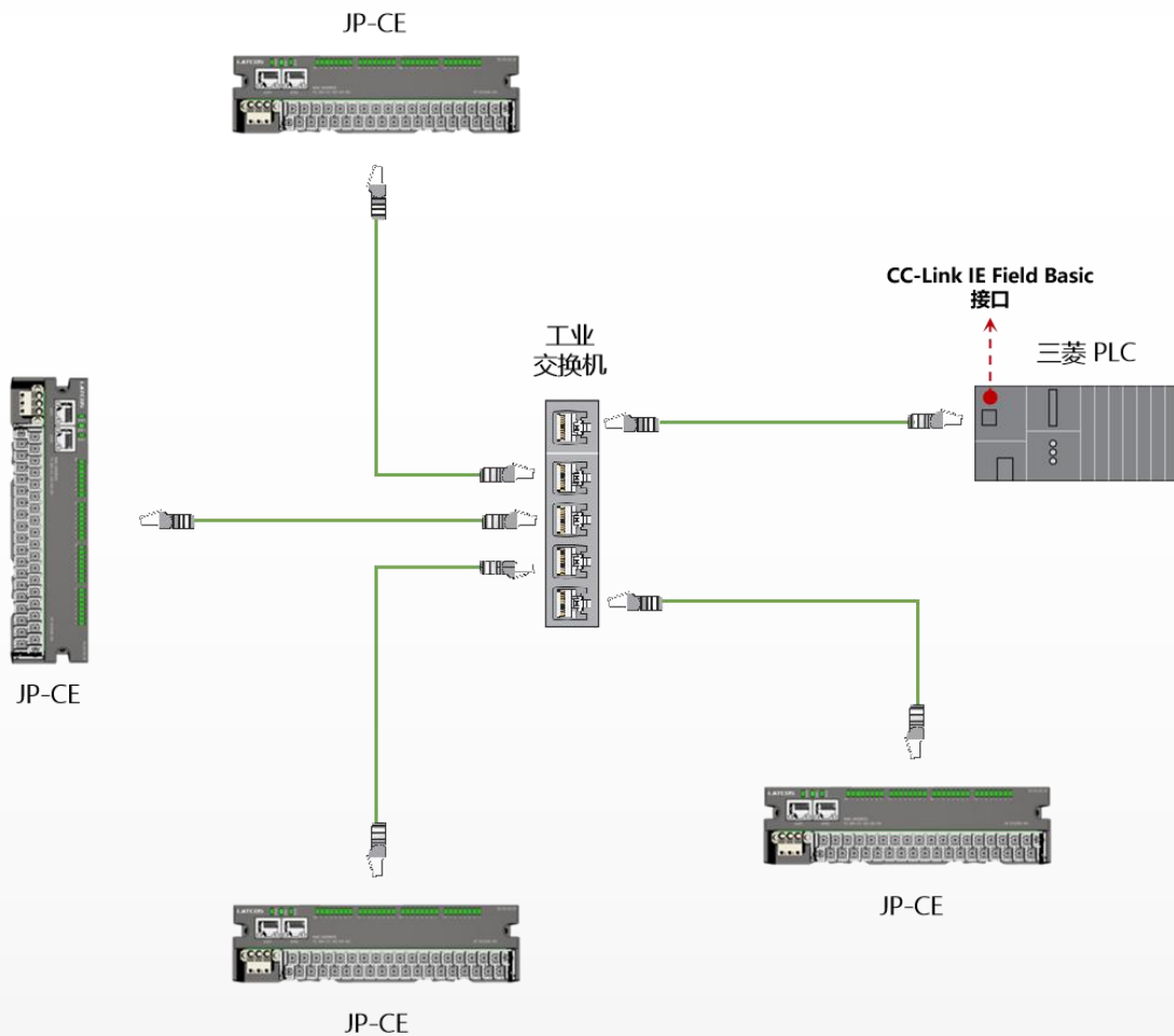
图 5-1 CC-Link IE Field Basic 星型网络拓扑结构
