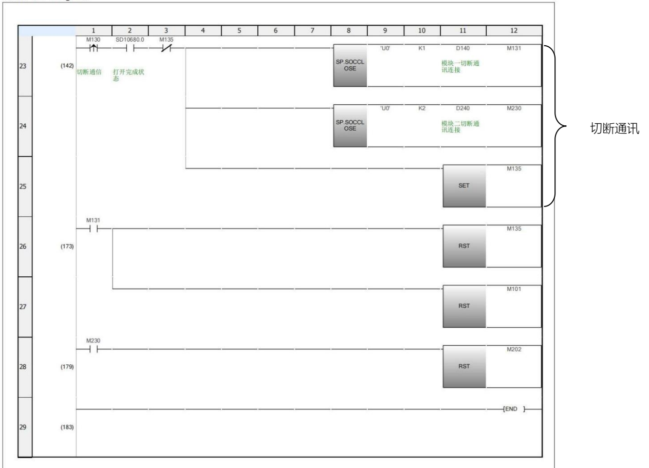
梯形图 数据名：ProgPou
